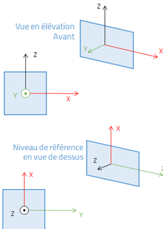
Fig. 17 - Axes de référence
